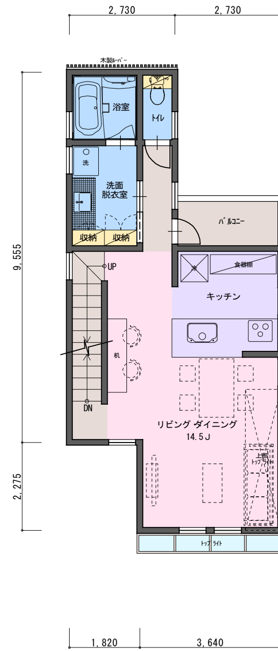
2階平面図 48.03m 2 (14.5坪)
