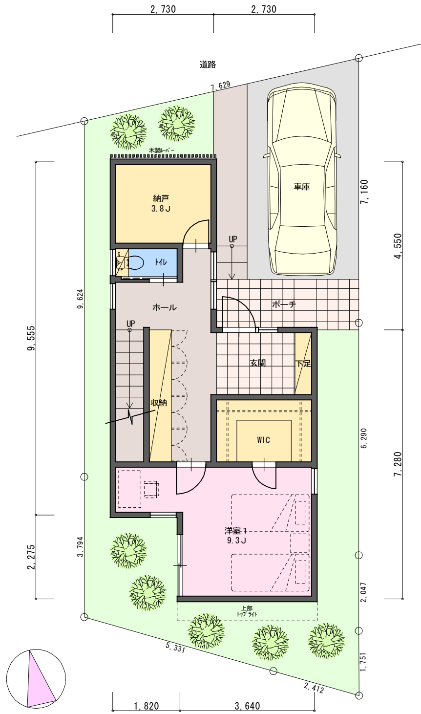
1階平面図 48.03m 2 (14.5坪)
